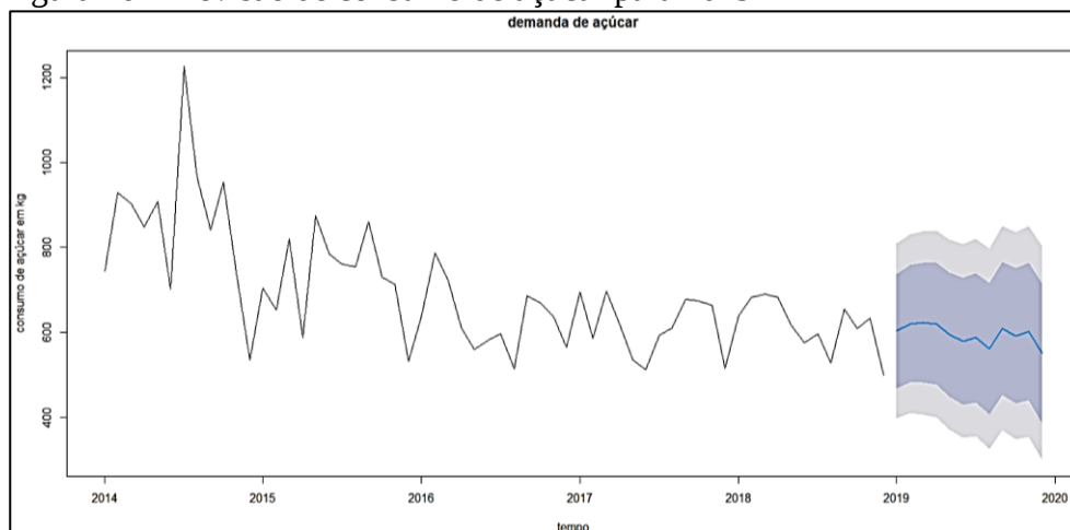
Figura 16 - Previsão de consumo de açúcar para 2019
