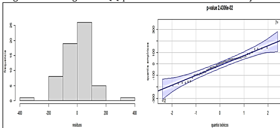
Figura 10 - Histograma e QQ-plot dos resíduos do modelo – açúcar
