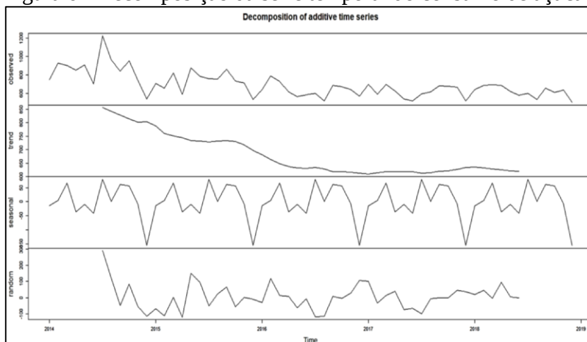
Figura 6 - Decomposição da série temporal do consumo de açúcar
