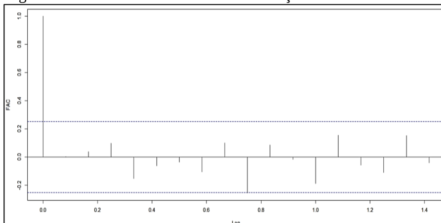
Figura 11 - FAC dos resíduos do modelo - açúcar
