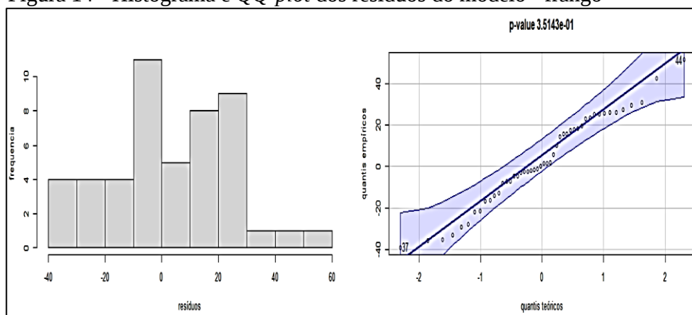
Figura 14 - Histograma e QQ-plot dos resíduos do modelo - frango
