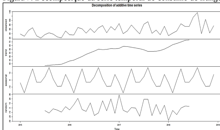
Figura 7. Decomposição da série temporal do consumo de frango
