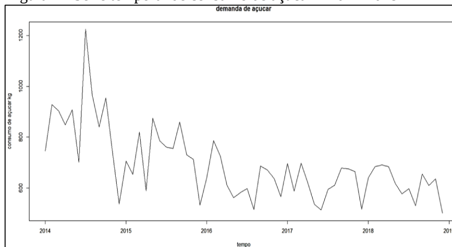
Figura 4 - Série temporal de consumo de açúcar – 2014-2018
