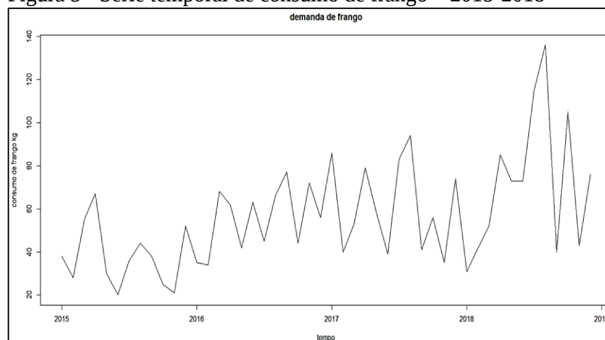
Figura 5 - Série temporal de consumo de frango – 2015-2018
