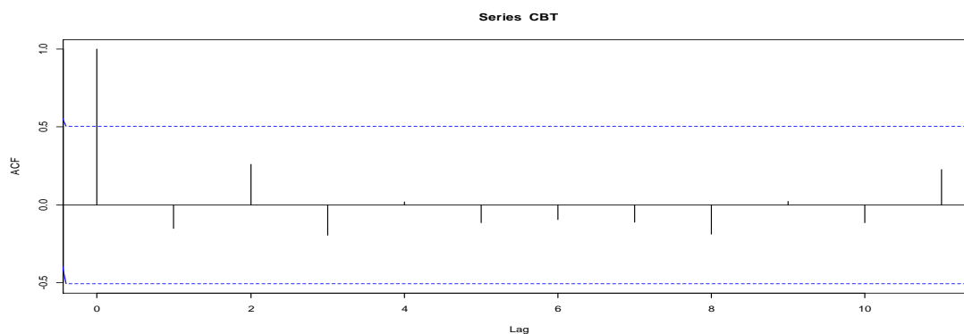
Figura 3 – Correlograma para CBT dos 15 meses em estudo
