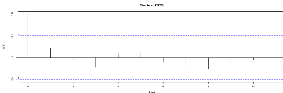
Figura 2 – Correlograma para CCS dos 15 meses em estudo
