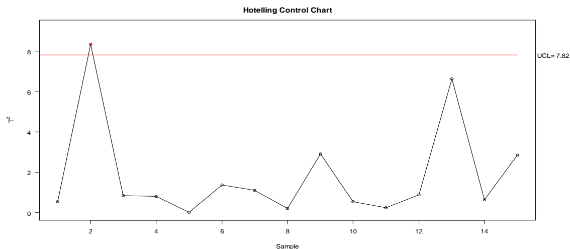
Figura 4 - Gráfico T^2 de Hotelling para CCS e CBT dos 15 meses em estudo, com \alpha = 5\% , fase .
