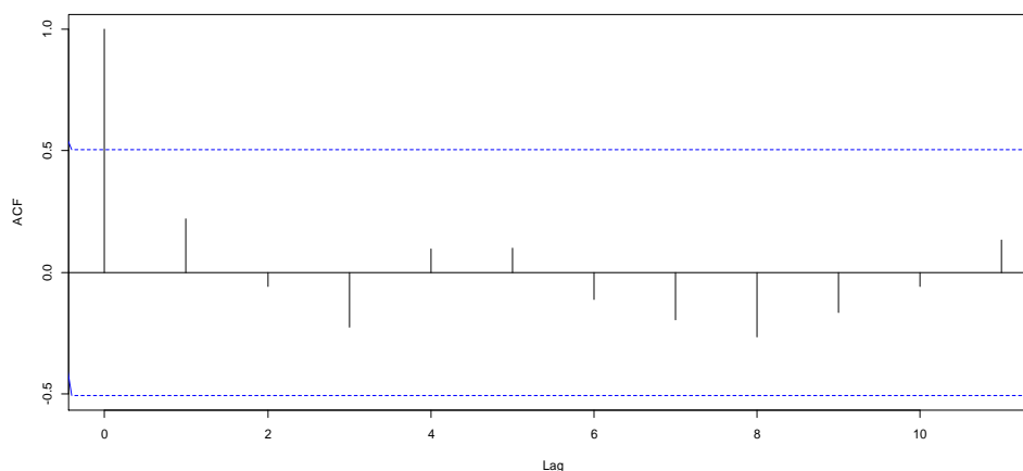
Figura 1 – Exemplo de Correlograma
