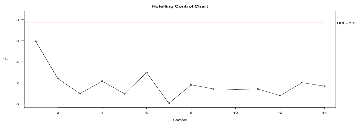
Figura 5 - Gráfico T^2 de Hotelling para CCS e CBT, com \alpha=5\% , fase 1, sem amostra 2
